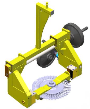
Lastaufnahmemittel Turbinenscheibe
