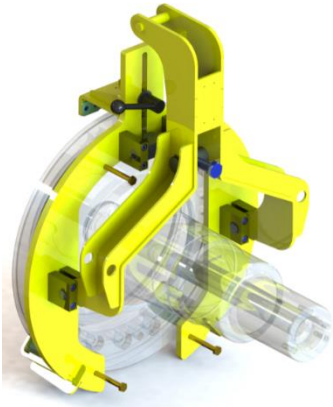
Lastaufnahmemittel Walzenstummel
